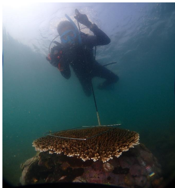
Gambar 2. Pengambilan Data Menggunakan Metode LIT
