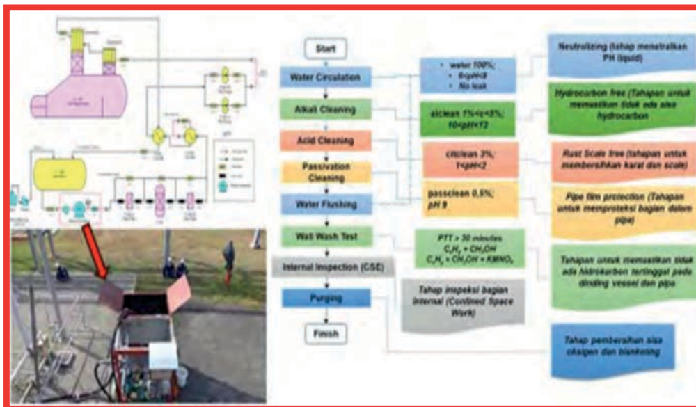
Gambar 86. Skema Inovasi Metode WASIAT
