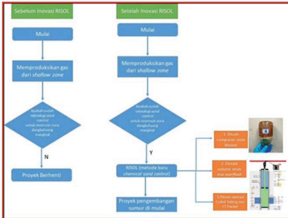
Gambar 74. Skema Penerapan Inovasi RISOL
