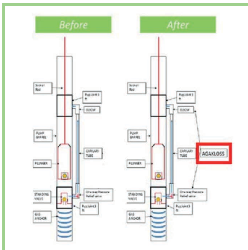
Gambar 92. Perbandingan Sebelum dan Sesudah Penerapan Inovasi AGAKLOSS
