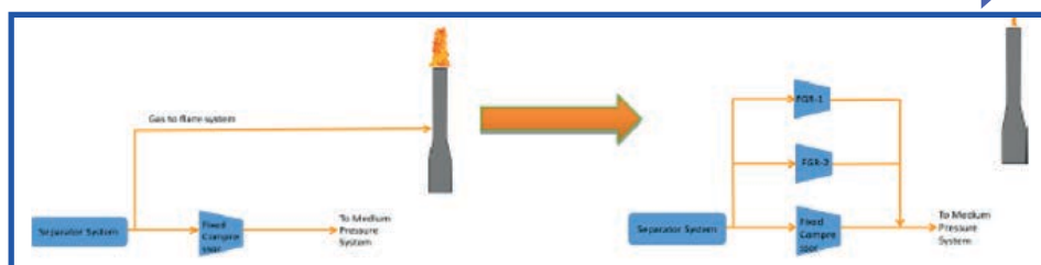
Gambar 52. Perbedaan system Sebelum dan Sesudah Penerapan Inovasi FGR
