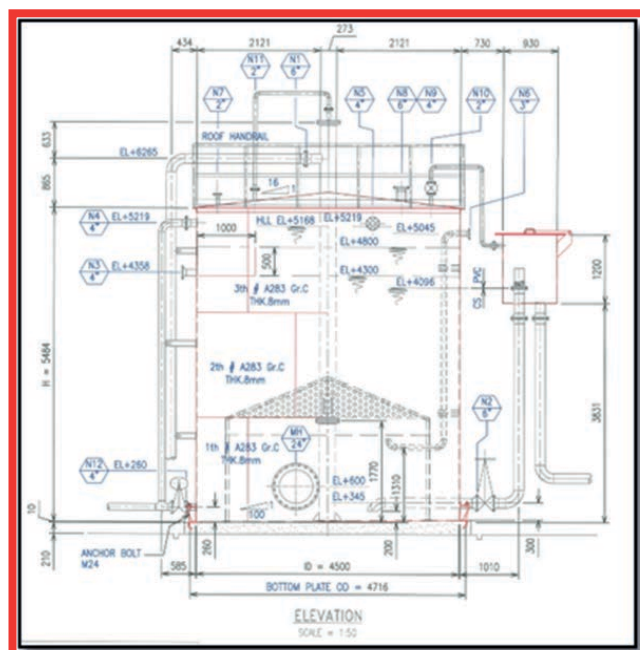
Gambar 61. Skema Inovasi Redesign Storage Tank di SPU VI TLJ
