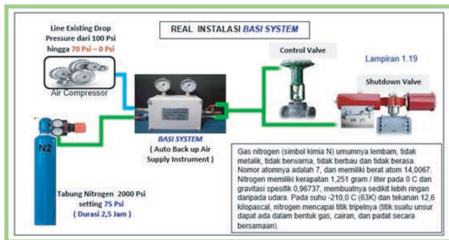
Gambar 14. Skema Inovasi Efisiensi Energi BASI System
