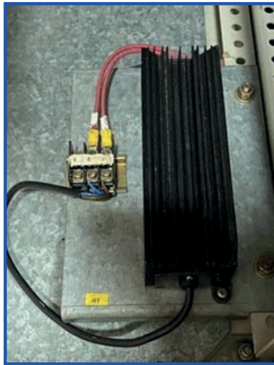
Gambar 39. Modifikasi HVAC Switchgear Panel di MCC Heater
