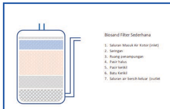
Gambar 182. Perangkat Biosand Filter
