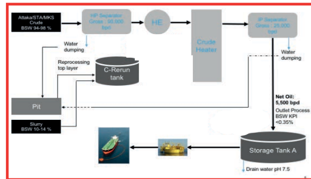
Gambar 82. Skema Proses Sebelum Program ADEM
