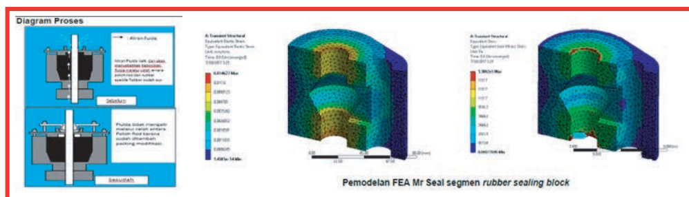
Gambar 65. Alur Proses dan Pemodelan Mister Sealer
