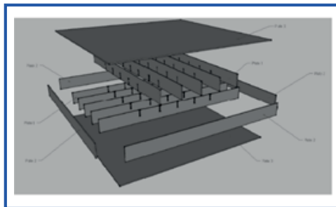
Gambar 38. Ilustrasi Struktur Waffle Crane Mat
