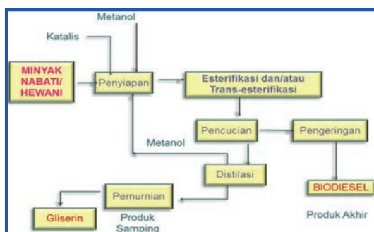
Gambar 41. Skema Inovasi Biodiesel B30
