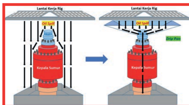
Gambar 58. Ilustrasi Aplikasi DRIP PAN
