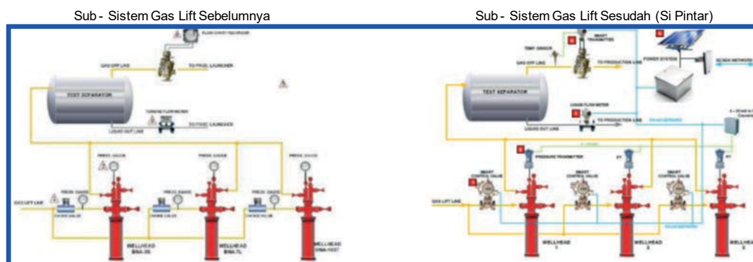
Gambar 43. Perubahan Skema Sistem Gas Setelah Penerapan Inovasi SIPINTAR
