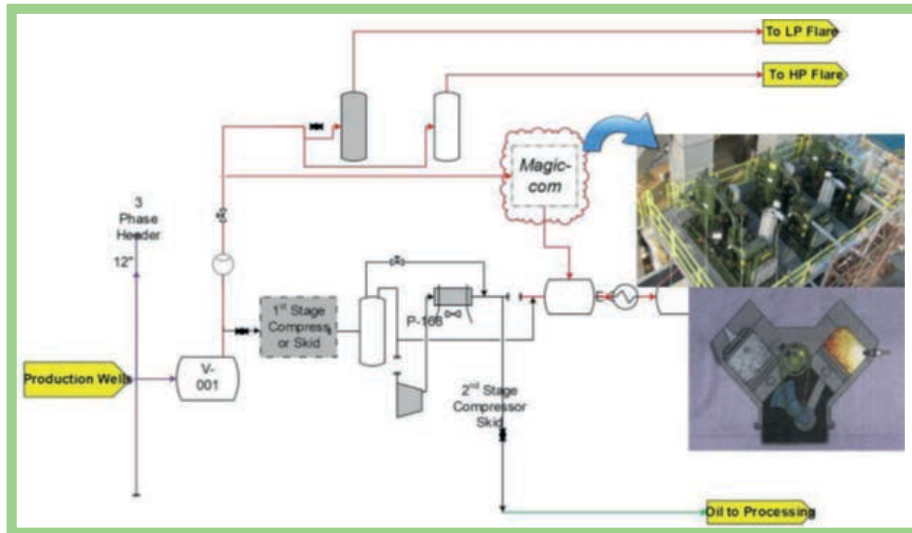
Gambar 15. Skema Inovasi MAGIC-COM
