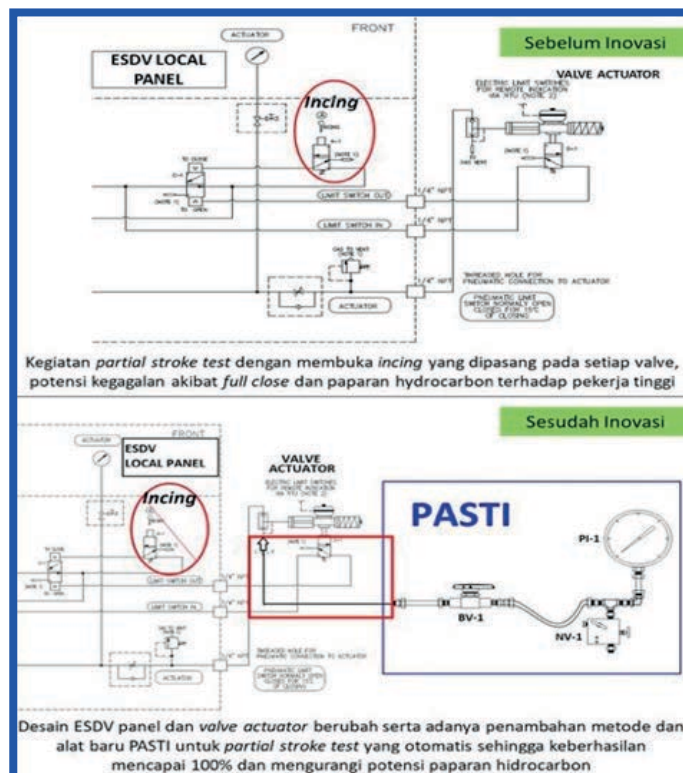
Gambar 45. Perbedaan Sistem Sebelum dan Sesudah Penerapan Inovasi PASTI
