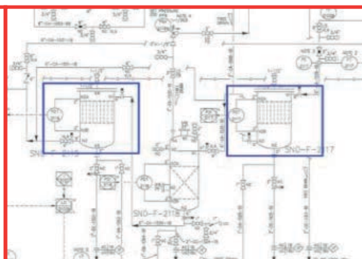
Gambar 88. Marked-up P&ID Modifikasi Pengaturan DP High Alarm pada Sistem Filtrasi Amine
