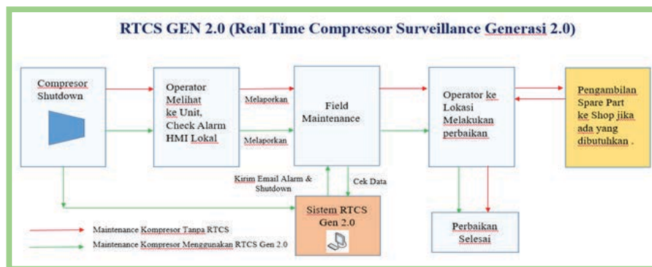
Gambar 27. Alur Perenapan Modifikasi RTCS Gen 2.0)
