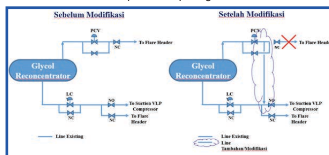
Gambar 53. Perbedaan sebelum dan setelah penerapan modifikasi LEBAR
