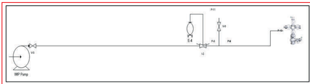
Gambar 125. Sketsa Proses Injeksi Chemical Asam Menggunakan Valve Ventury
