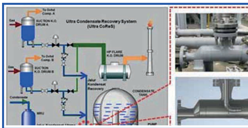
Gambar 37. Skema Proses Setelah Penambahan ICOMS
