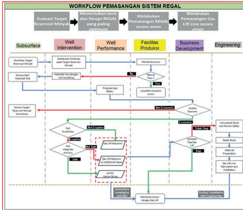
Gambar 131. Skema Program Inovasi REGAL
