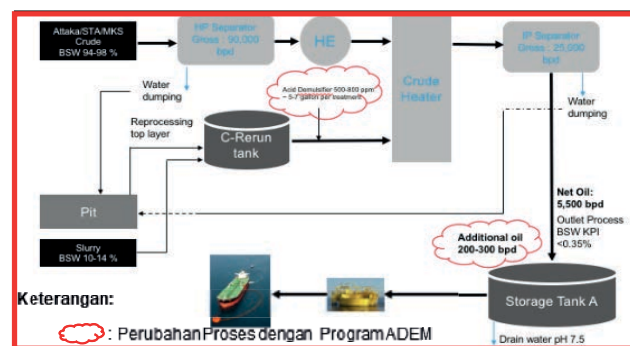
Gambar 83. Skema Proses Setelah Program ADEM
