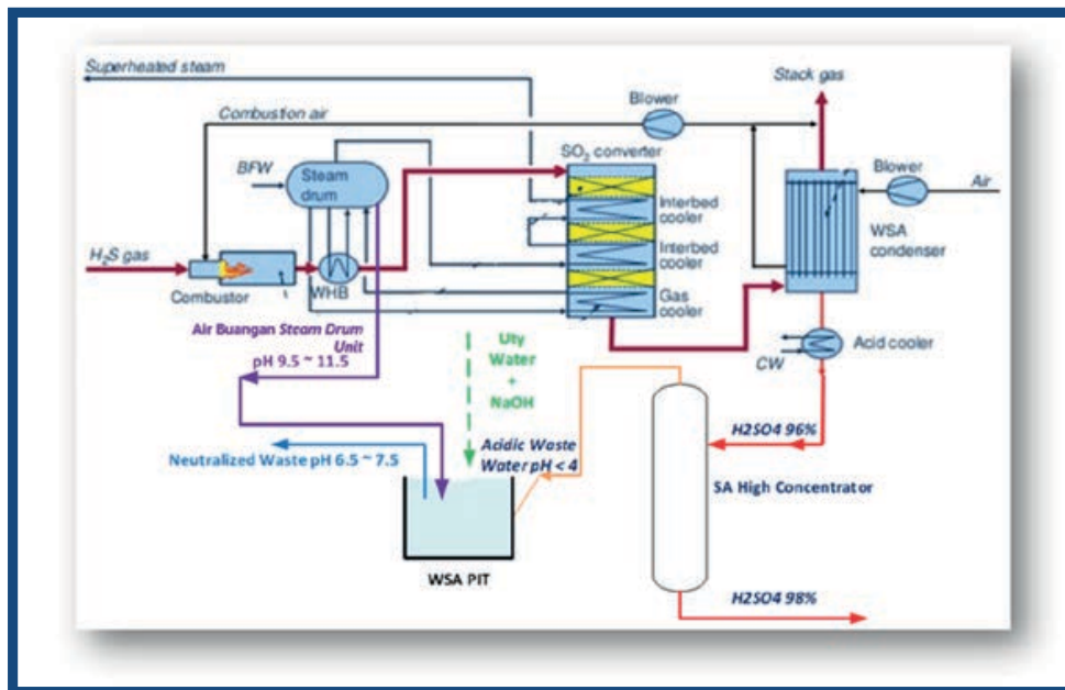
Gambar 121. Skema Modifikasi Proses Netralisasi Air Buangan di WSA Pit Menggunakan Air Buangan Steam Drum Unit
