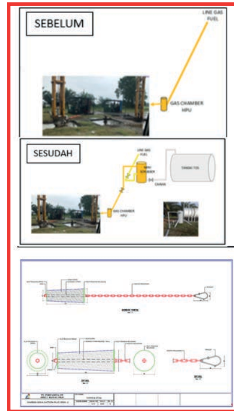
Gambar 57. Perbandingan Sebelum dan Setelah Inovasi Section Plug
