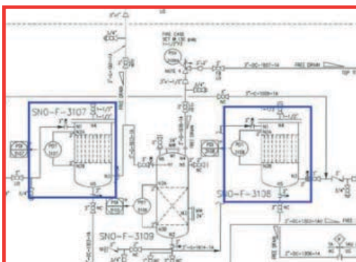
Gambar 87. Marked-up P&ID modifikasi Pengaturan DP High Alarm pada Sistem Filtrasi TEG
