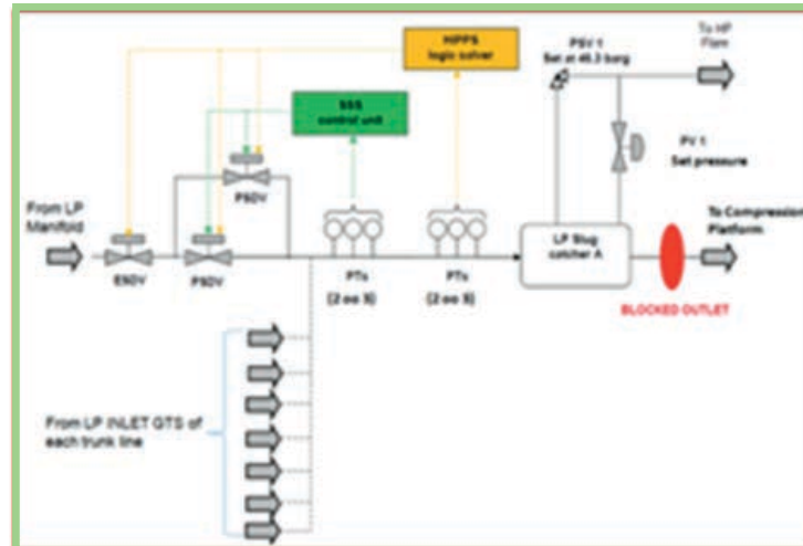
Gambar 22. Skema Inovasi ZOMBIE
