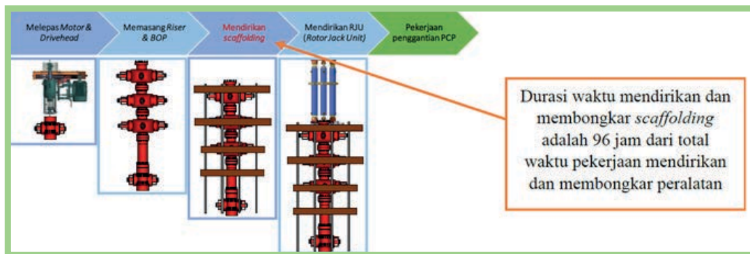
Gambar 28. Alur Pekerjaan Mendirikan Unit untuk Reaktivasi Sumur PCP dengan Scaffolding
